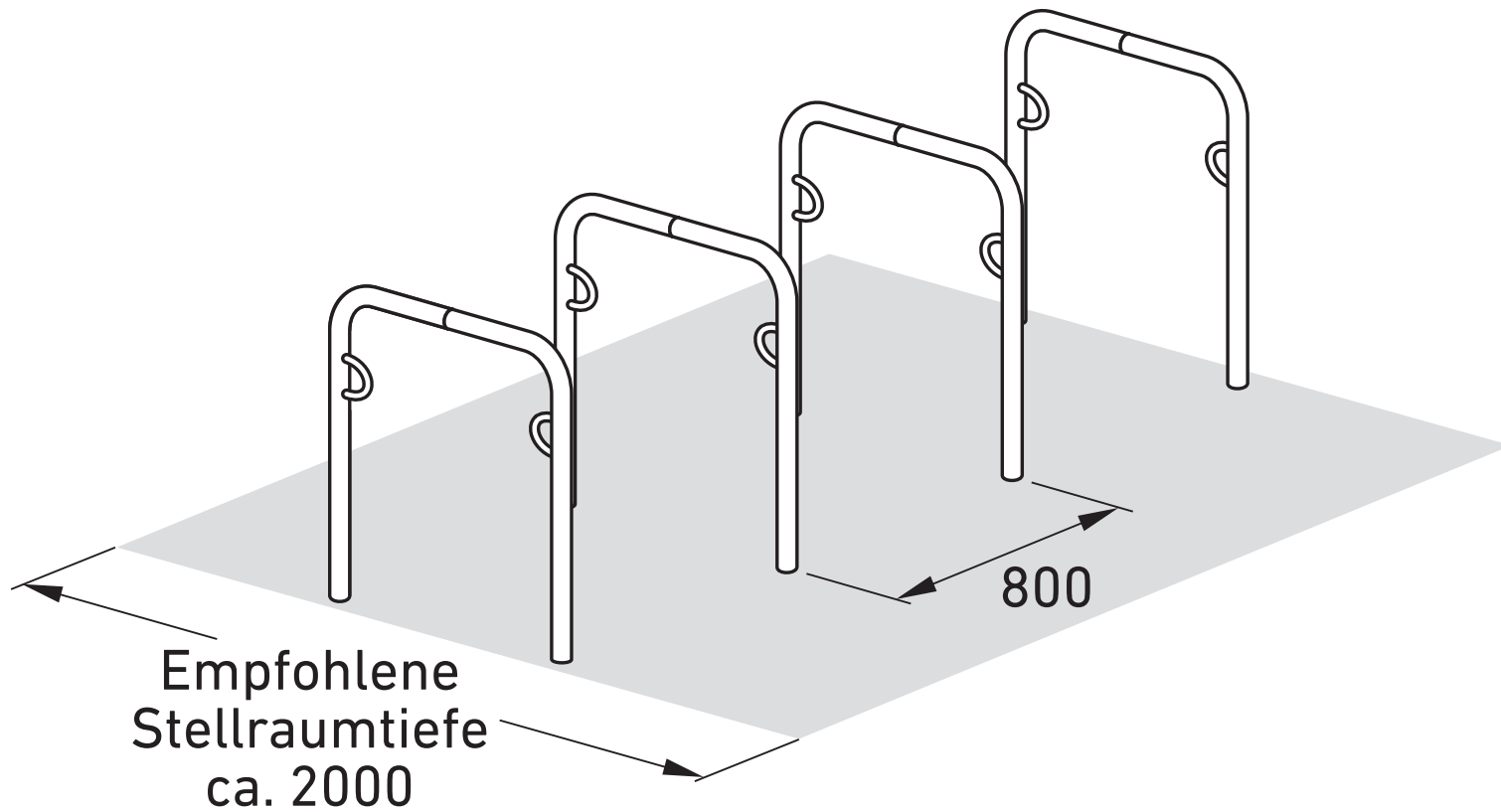
Profondeur de l'espace de stationnement recommandé
